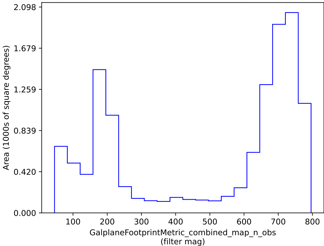
baseline_v3.3_10yrs : GalplaneFootprintMetric_combined_map_n_obs
