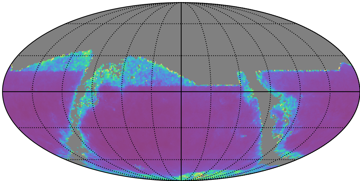
baseline_v3.3_10yrs z band: AGN SF_uncert
