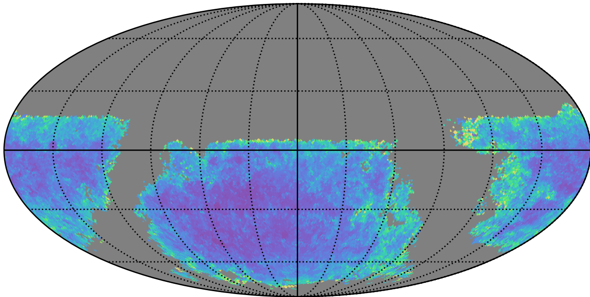
baseline_v3.3_10yrs u band: AGN SF_uncert
