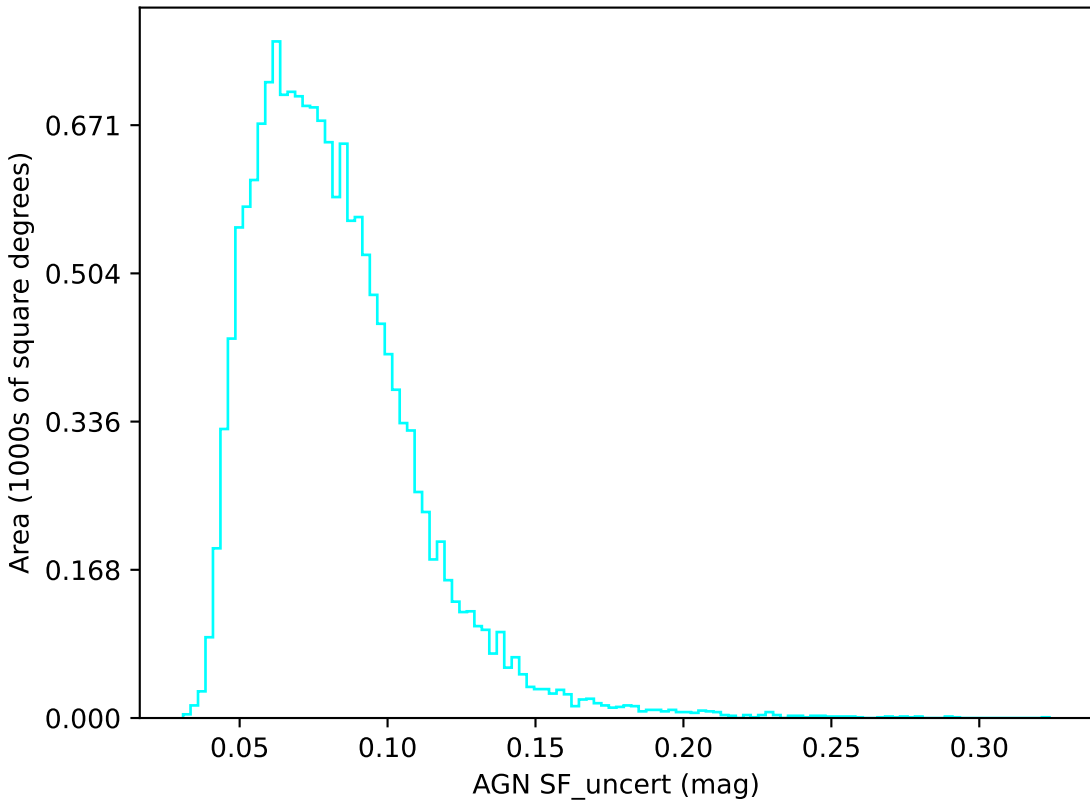
baseline_v3.3_10yrs u band: AGN SF_uncert
