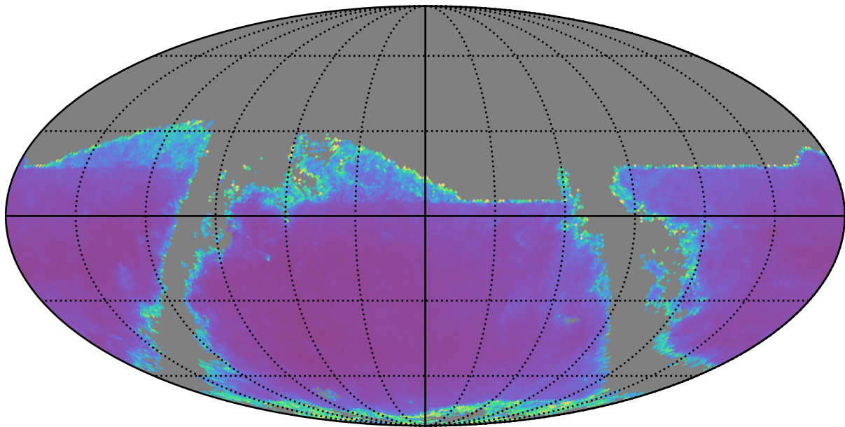
baseline_v3.3_10yrs r band: AGN SF_uncert
