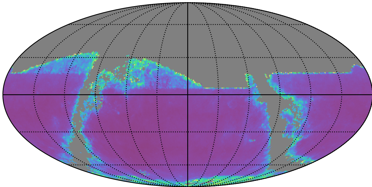
baseline_v3.3_10yrs i band: AGN SF_uncert
