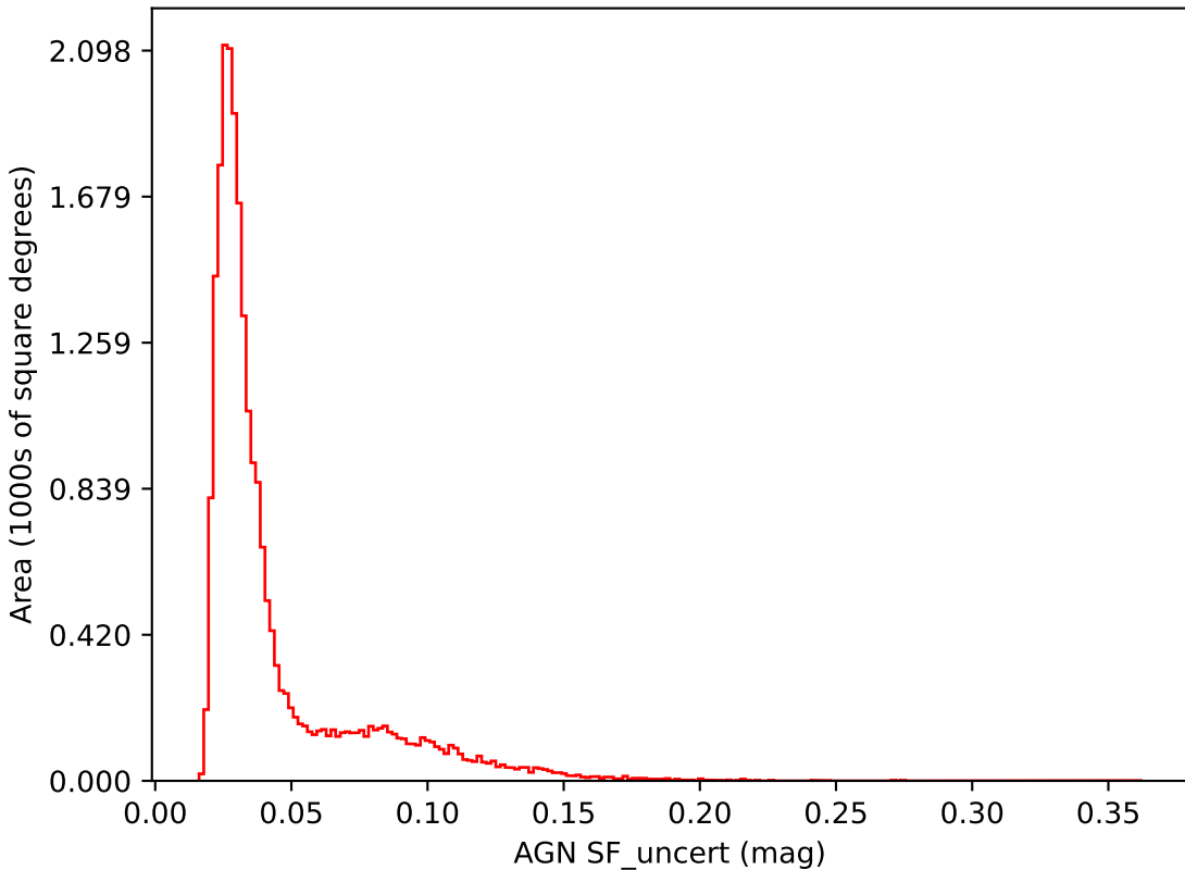
baseline_v3.3_10yrs i band: AGN SF_uncert
