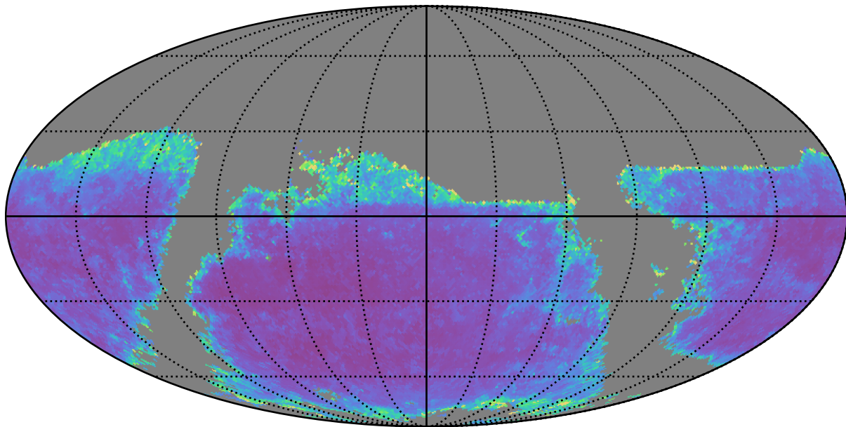
baseline_v3.3_10yrs g band: AGN SF_uncert
