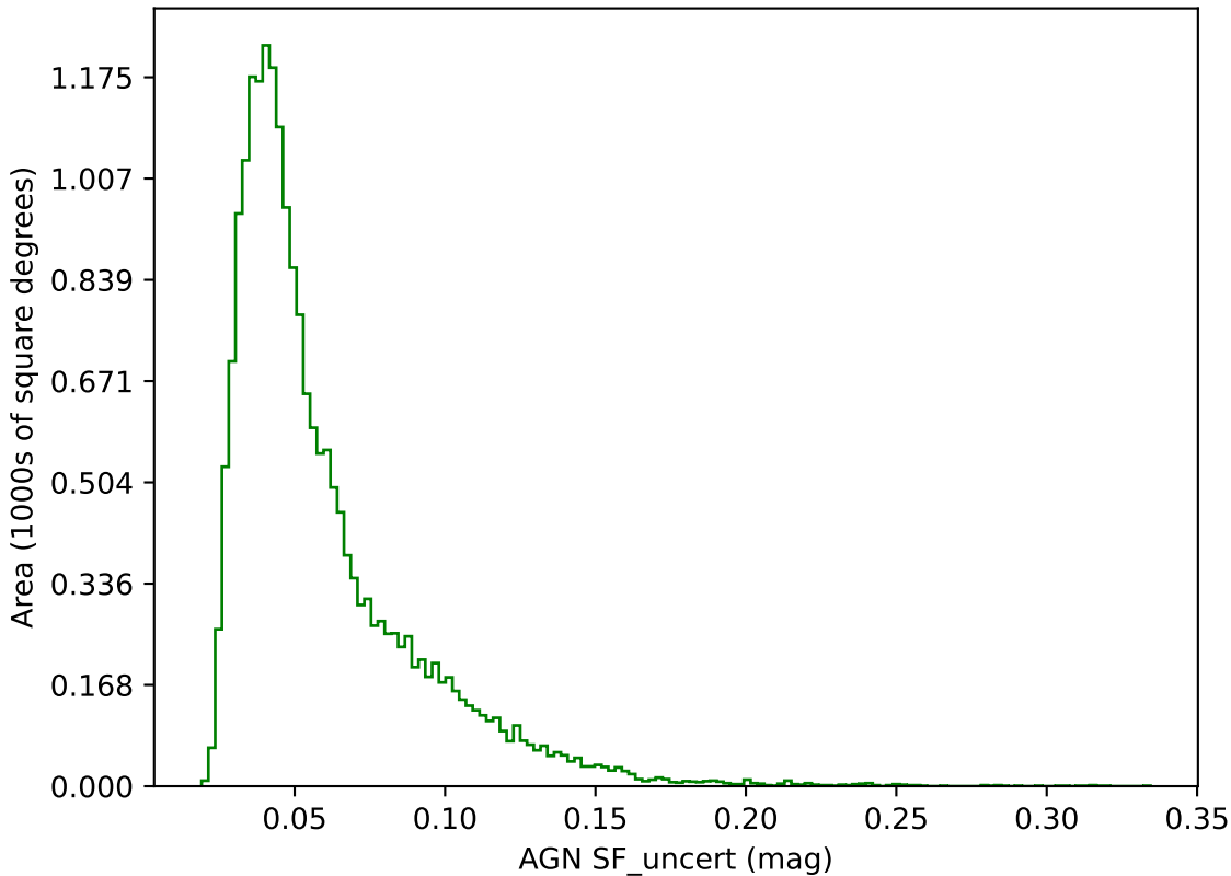
baseline_v3.3_10yrs g band: AGN SF_uncert
