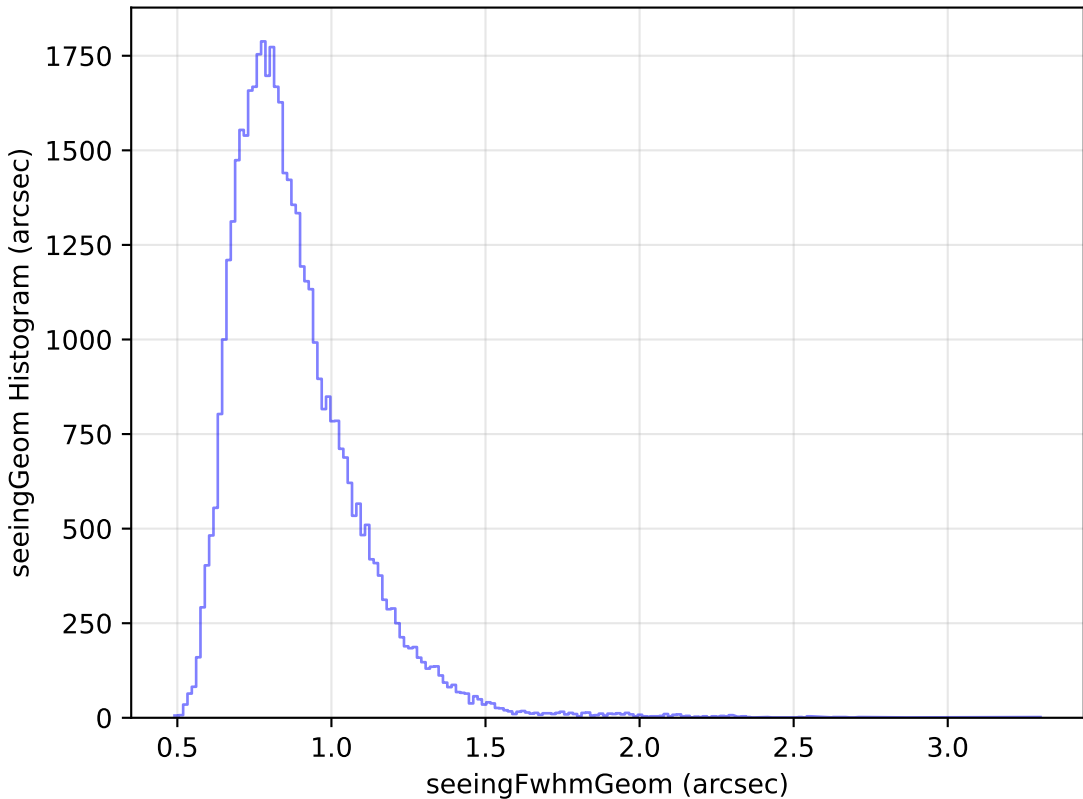
baseline_v3.3_10yrs Yr 1 y band: seeingGeom Histogram
