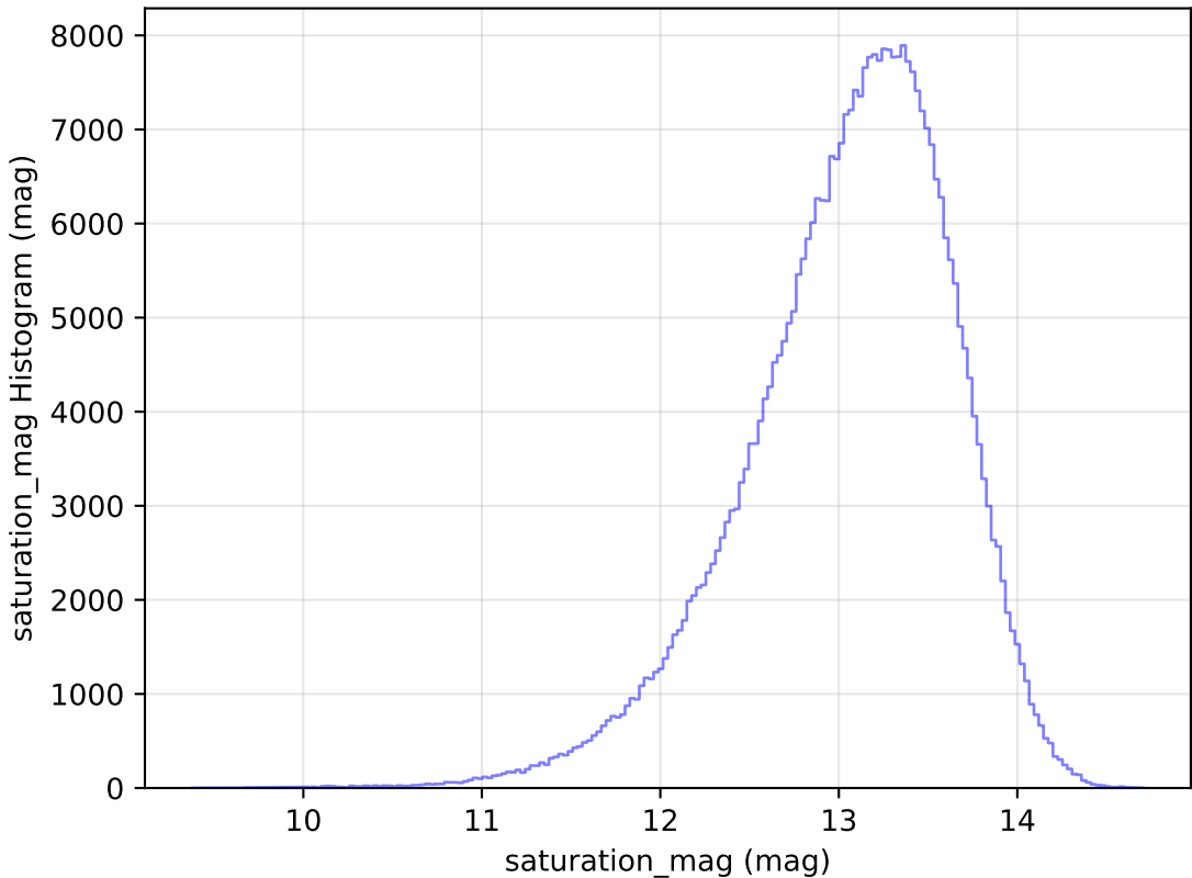
baseline_v3.3_10yrs All sky y band: saturation_mag Histogram
