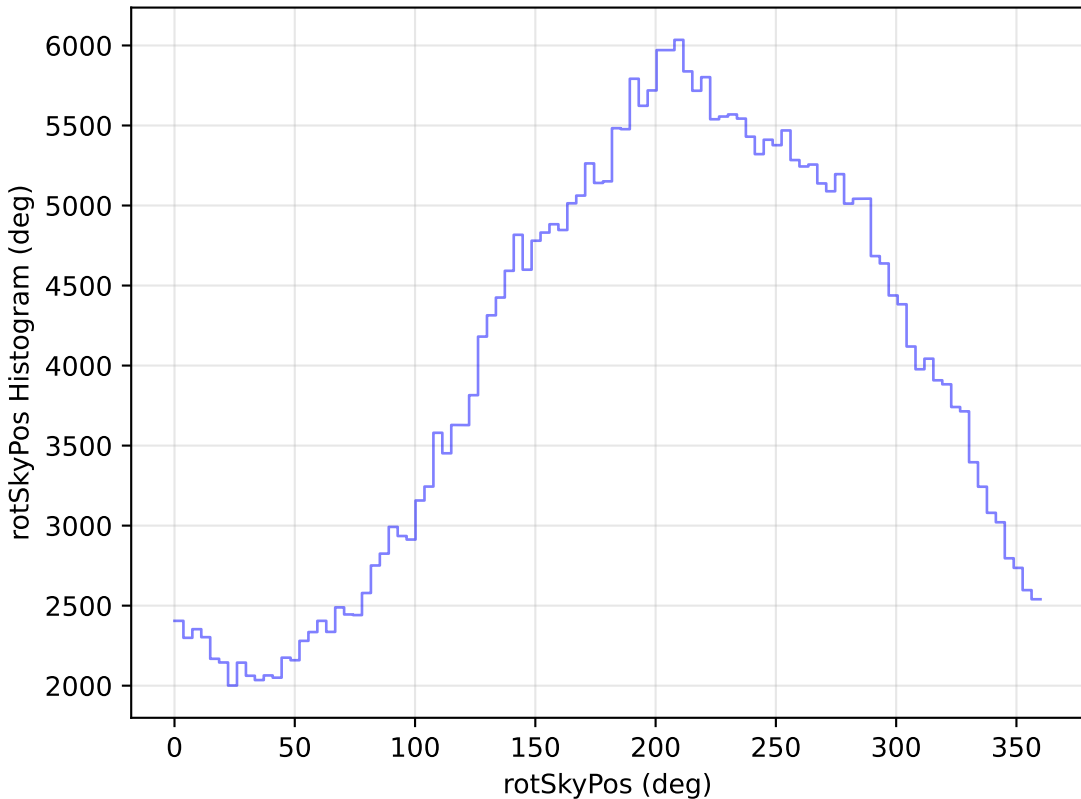
baseline_v3.3_10yrs WFD y band: rotSkyPos Histogram
