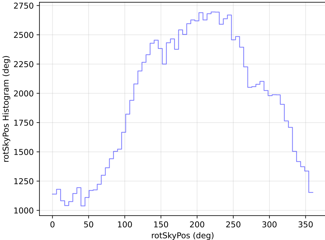
baseline_v3.3_10yrs WFD u band: rotSkyPos Histogram
