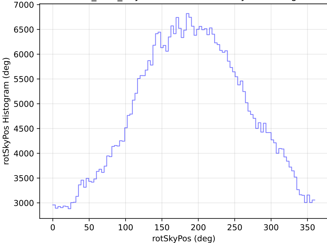
baseline_v3.3_10yrs WFD r band: rotSkyPos Histogram
