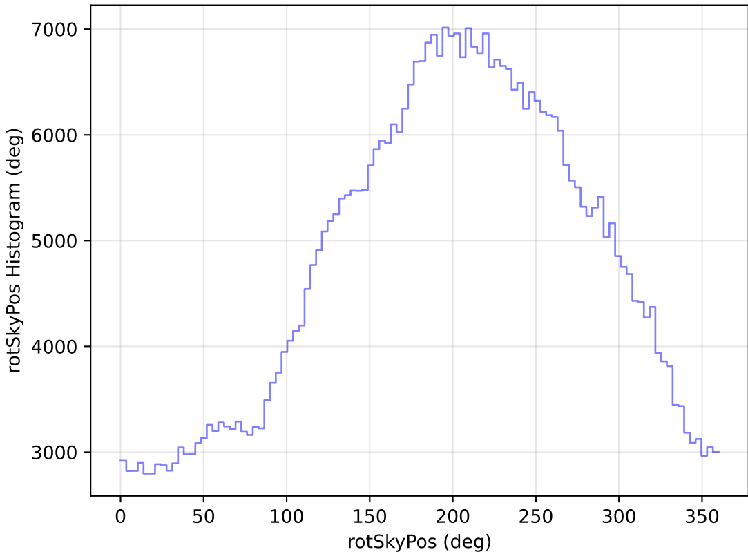
baseline_v3.3_10yrs WFD i band: rotSkyPos Histogram
