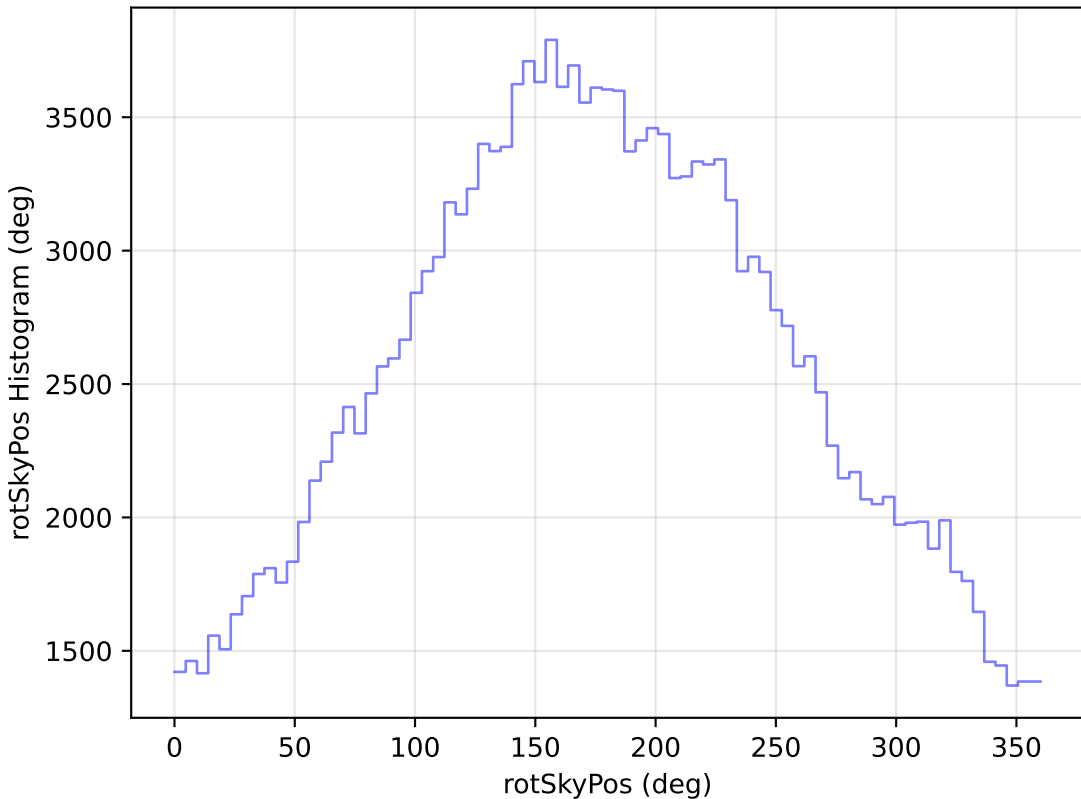
baseline_v3.3_10yrs WFD g band: rotSkyPos Histogram
