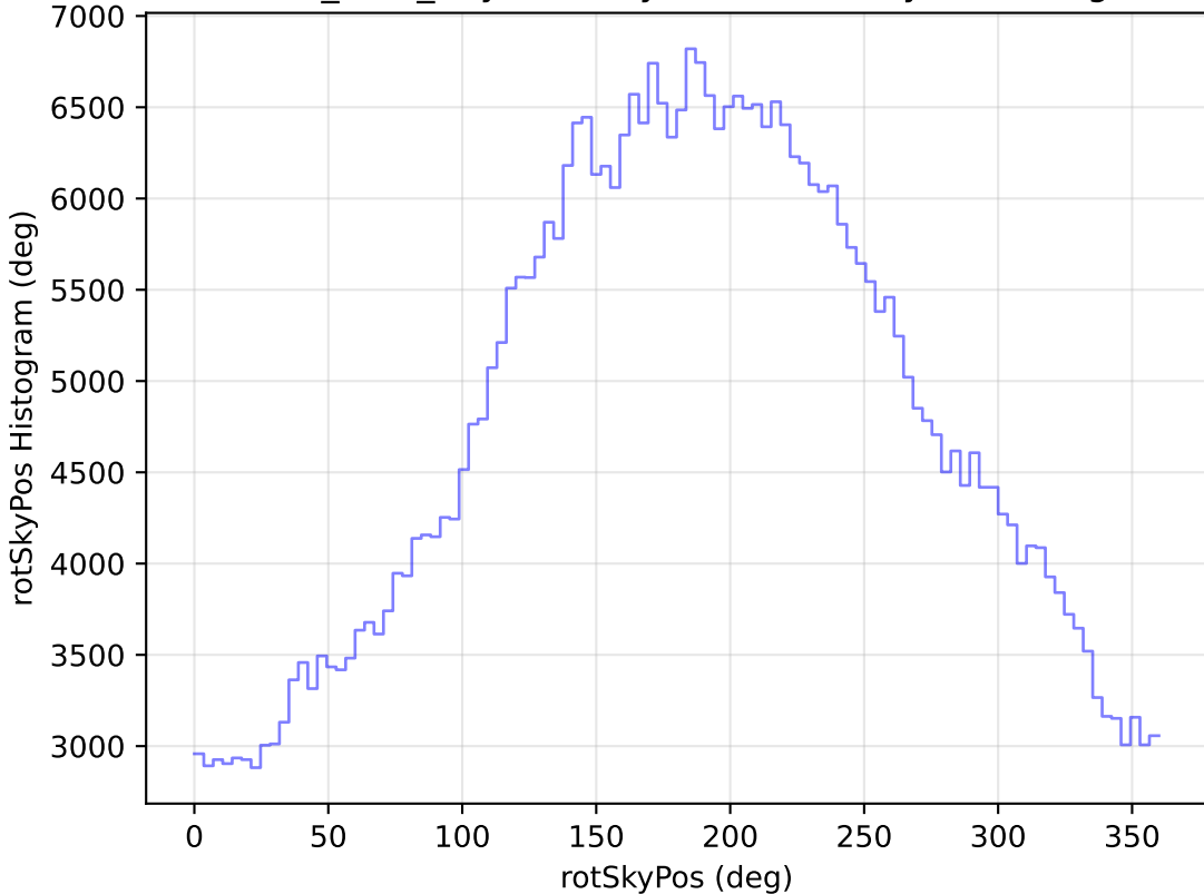
baseline_v3.3_10yrs All sky r band: rotSkyPos Histogram
