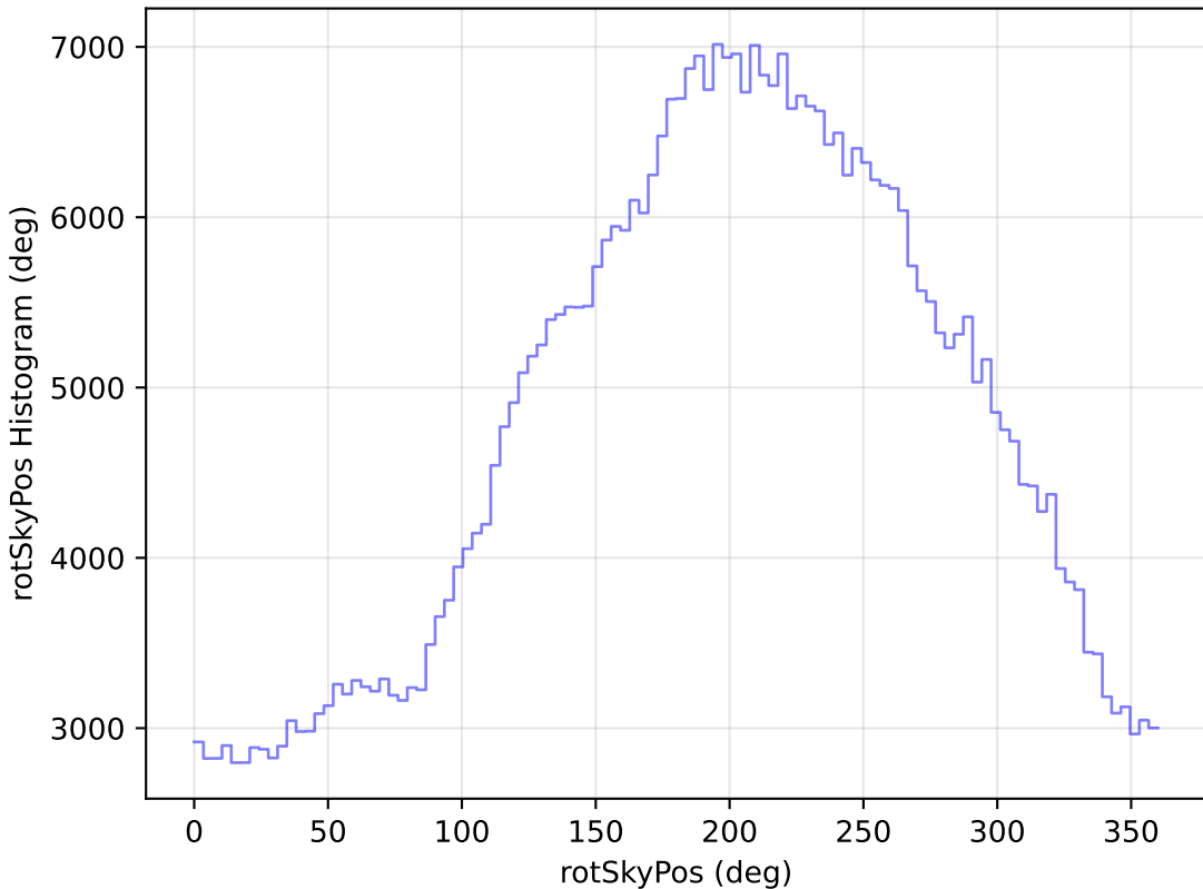
baseline_v3.3_10yrs All sky i band: rotSkyPos Histogram
