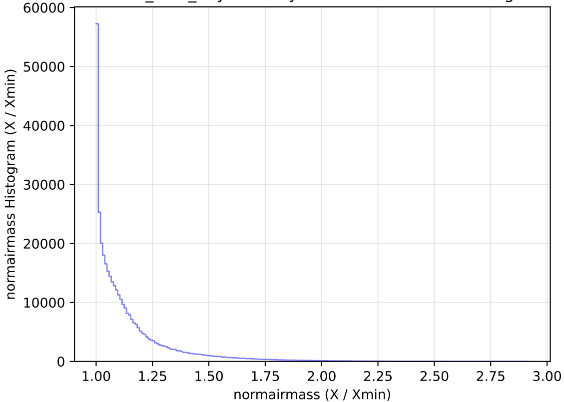
baseline_v3.3_10yrs WFD y band: normairmass Histogram
