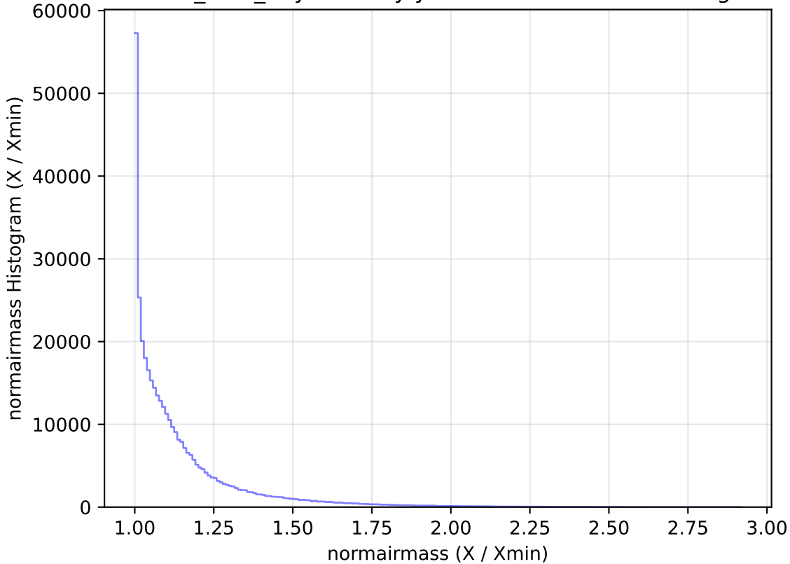
baseline_v3.3_10yrs All sky y band: normairmass Histogram
