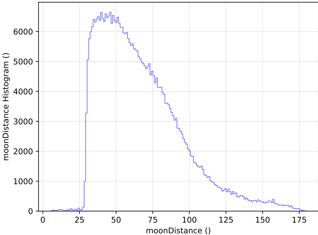
baseline_v3.3_10yrs WFD y band: moonDistance Histogram
