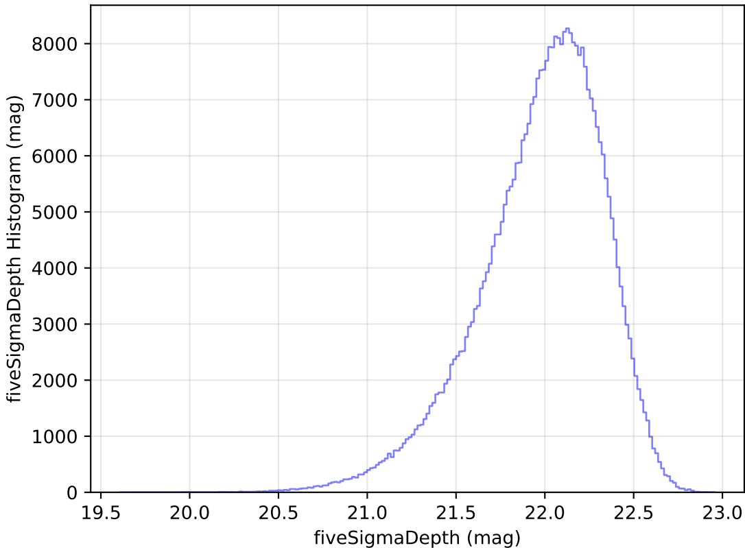
baseline_v3.3_10yrs WFD y band: fiveSigmaDepth Histogram
