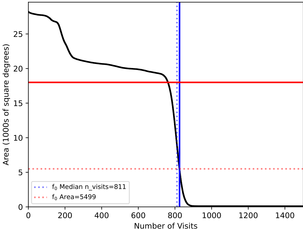
baseline_v3.3_10yrs All sky: f 0
