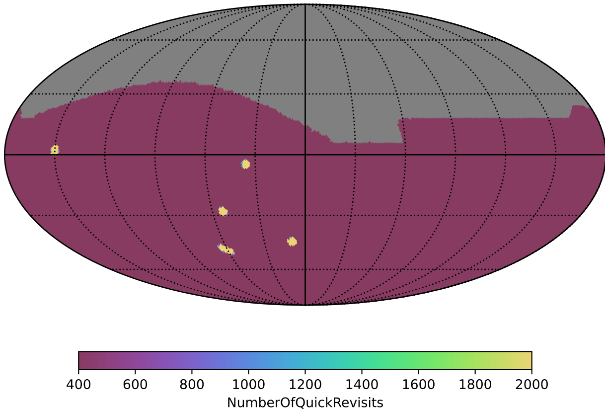
baseline_v3.3_10yrs All sky: NumberOfQuickRevisits
