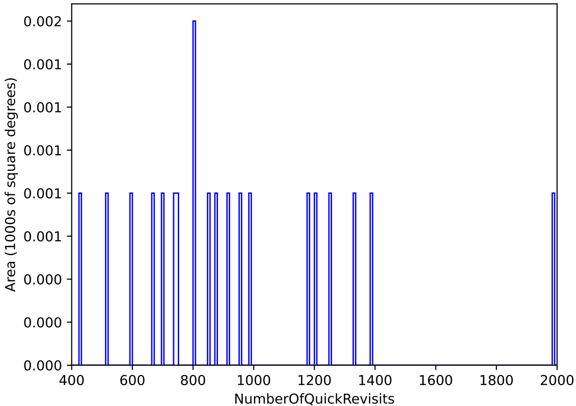
baseline_v3.3_10yrs All sky: NumberOfQuickRevisits
