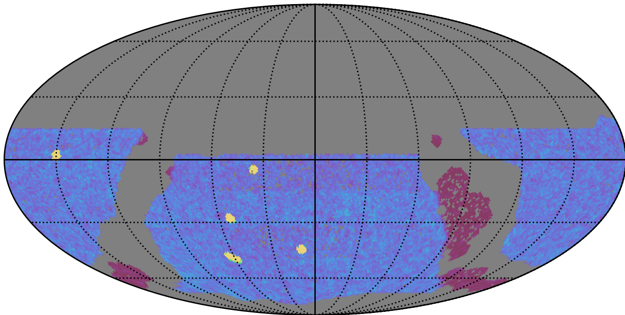
baseline_v3.3_10yrs WFD y band: NVisits
