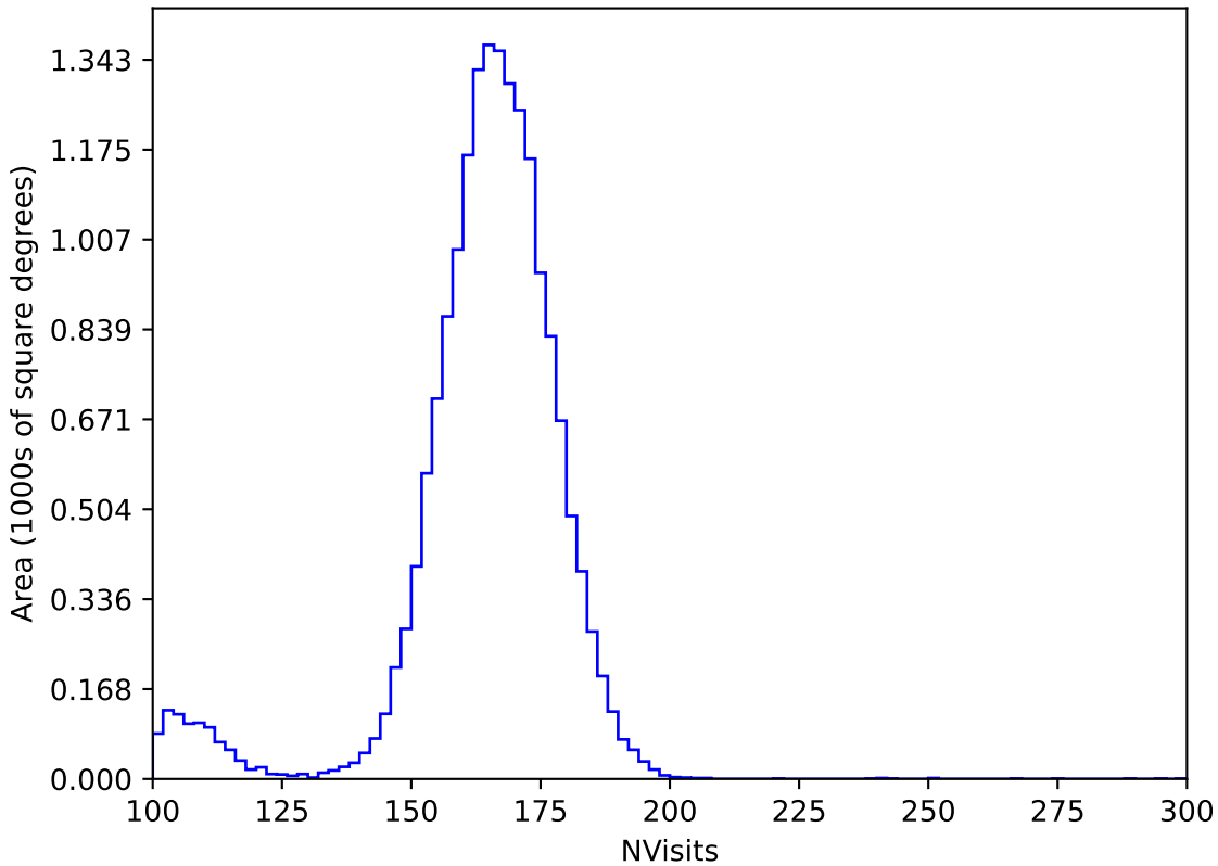
baseline_v3.3_10yrs WFD y band: NVisits
