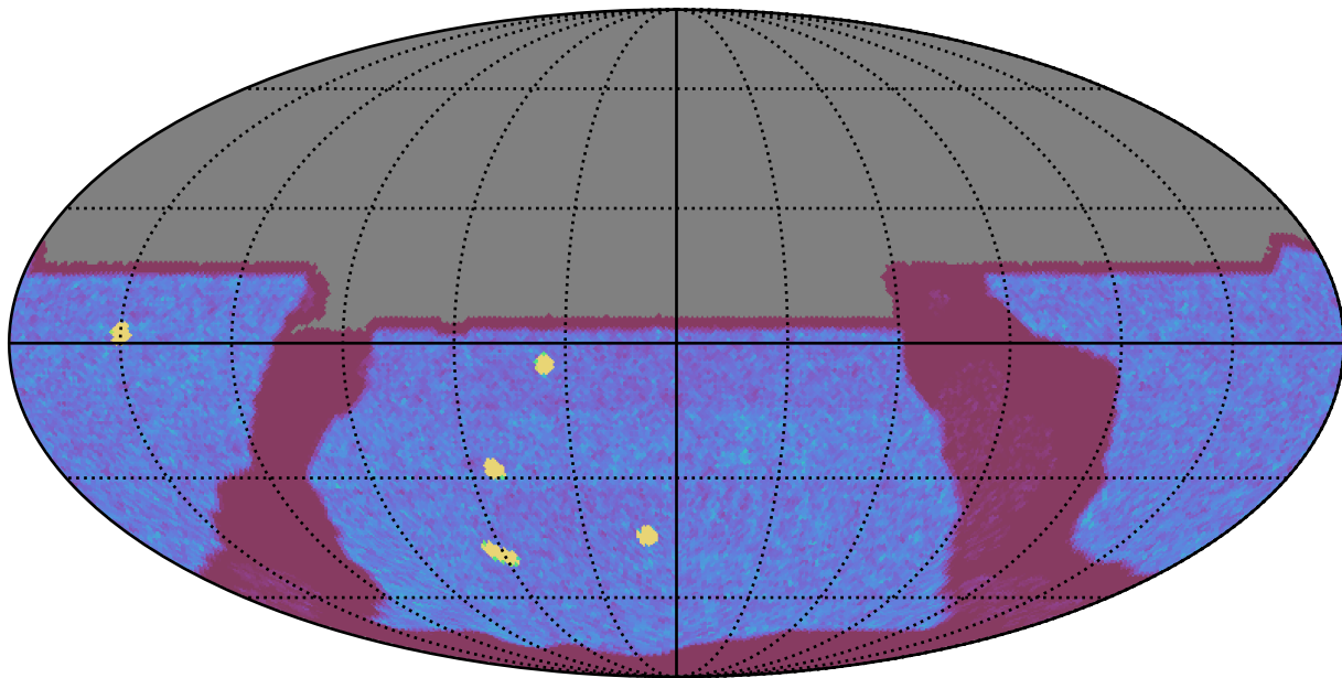
baseline_v3.3_10yrs All sky y band: NVisits
