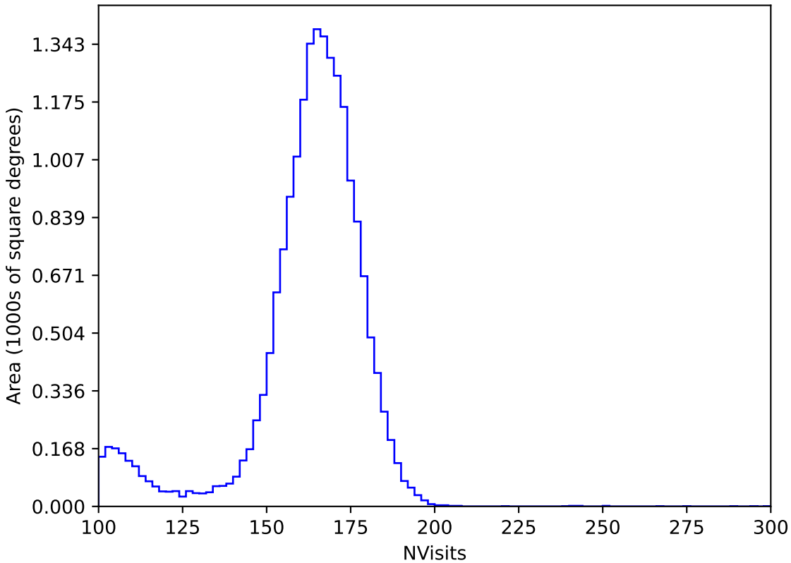
baseline_v3.3_10yrs All sky y band: NVisits
