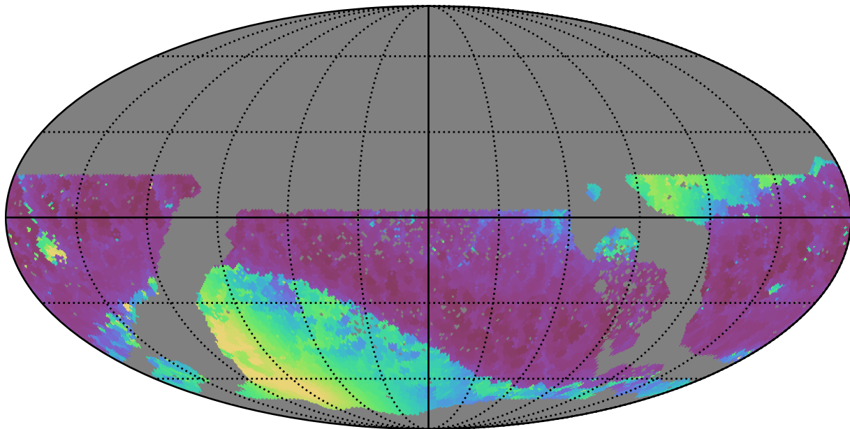
baseline_v3.3_10yrs WFD z band: Min solarElong
