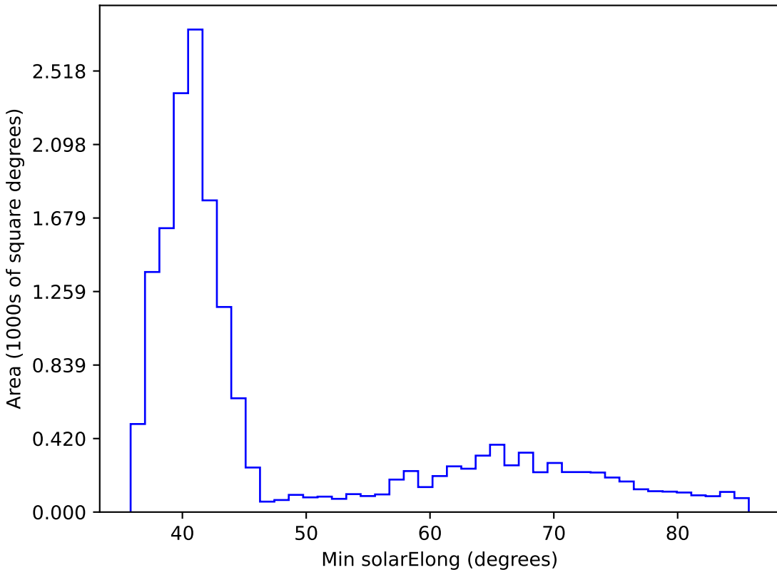
baseline_v3.3_10yrs WFD z band: Min solarElong
