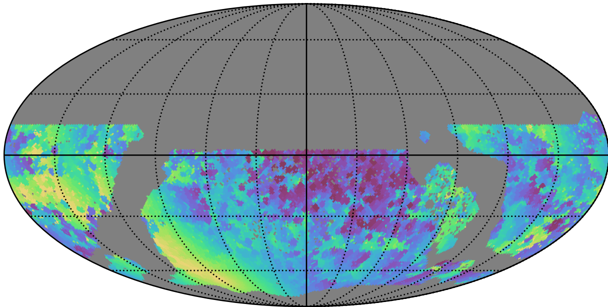
baseline_v3.3_10yrs WFD y band: Min solarElong
