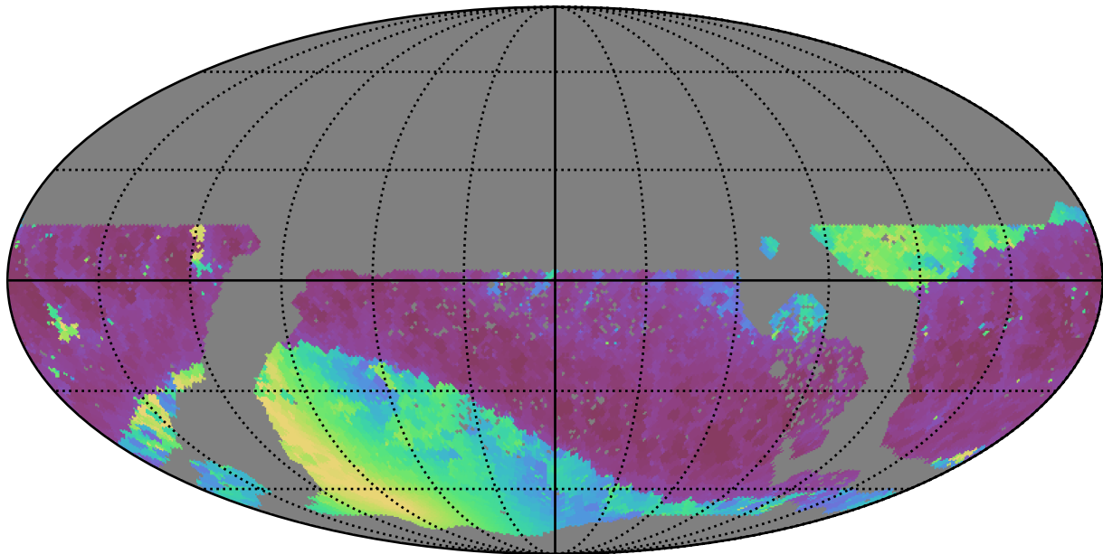
baseline_v3.3_10yrs WFD i band: Min solarElong
