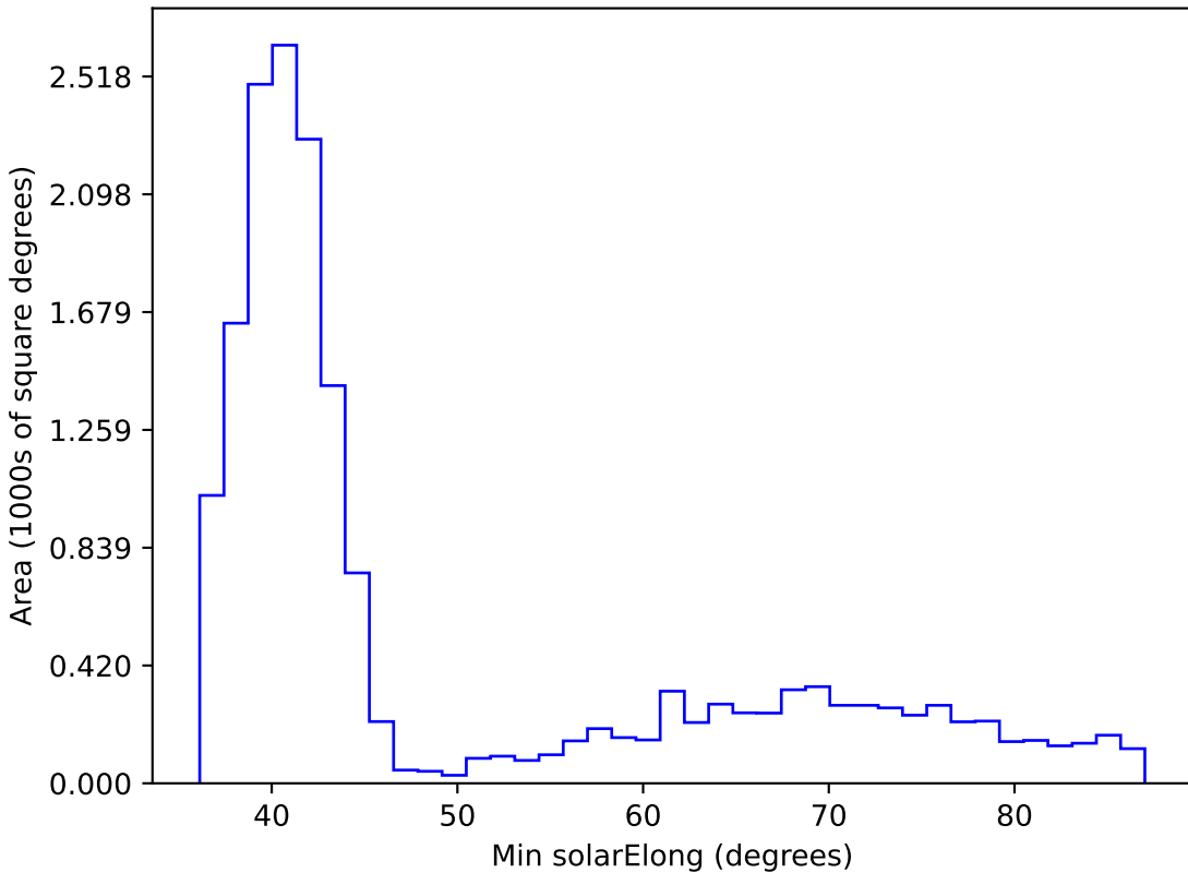
baseline_v3.3_10yrs WFD i band: Min solarElong
