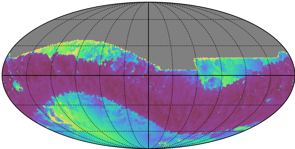
baseline_v3.3_10yrs All sky z band: Min solarElong
