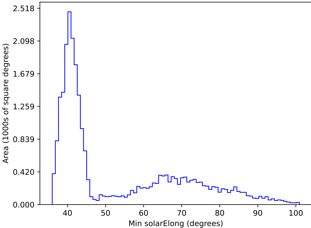
baseline_v3.3_10yrs All sky z band: Min solarElong
