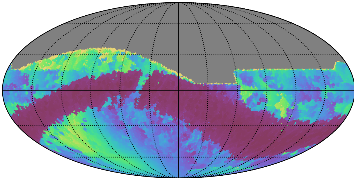
baseline_v3.3_10yrs All sky r band: Min solarElong
