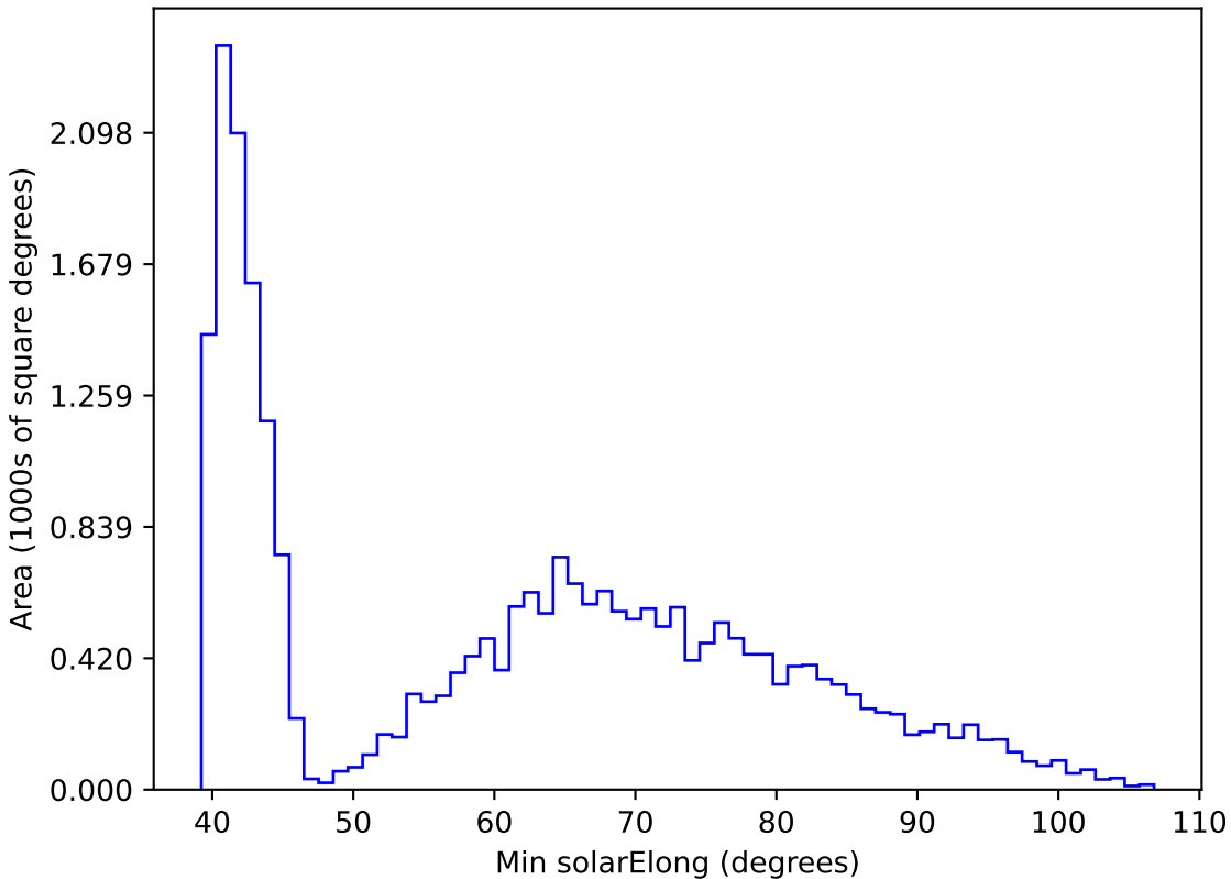
baseline_v3.3_10yrs All sky r band: Min solarElong
