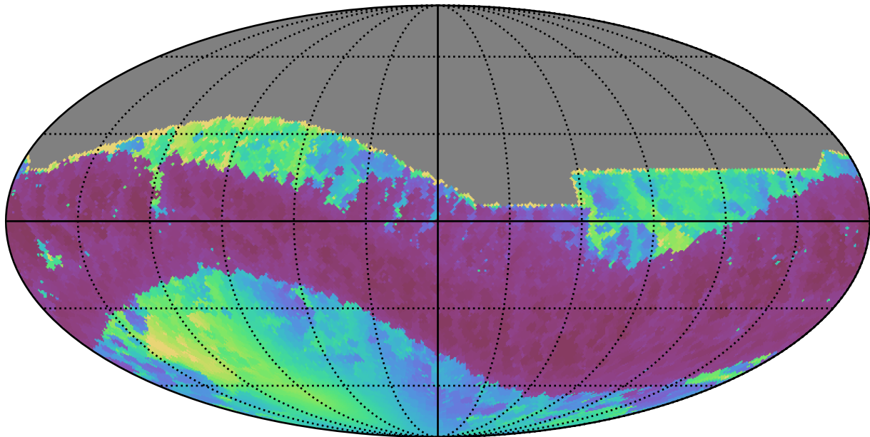
baseline_v3.3_10yrs All sky i band: Min solarElong
