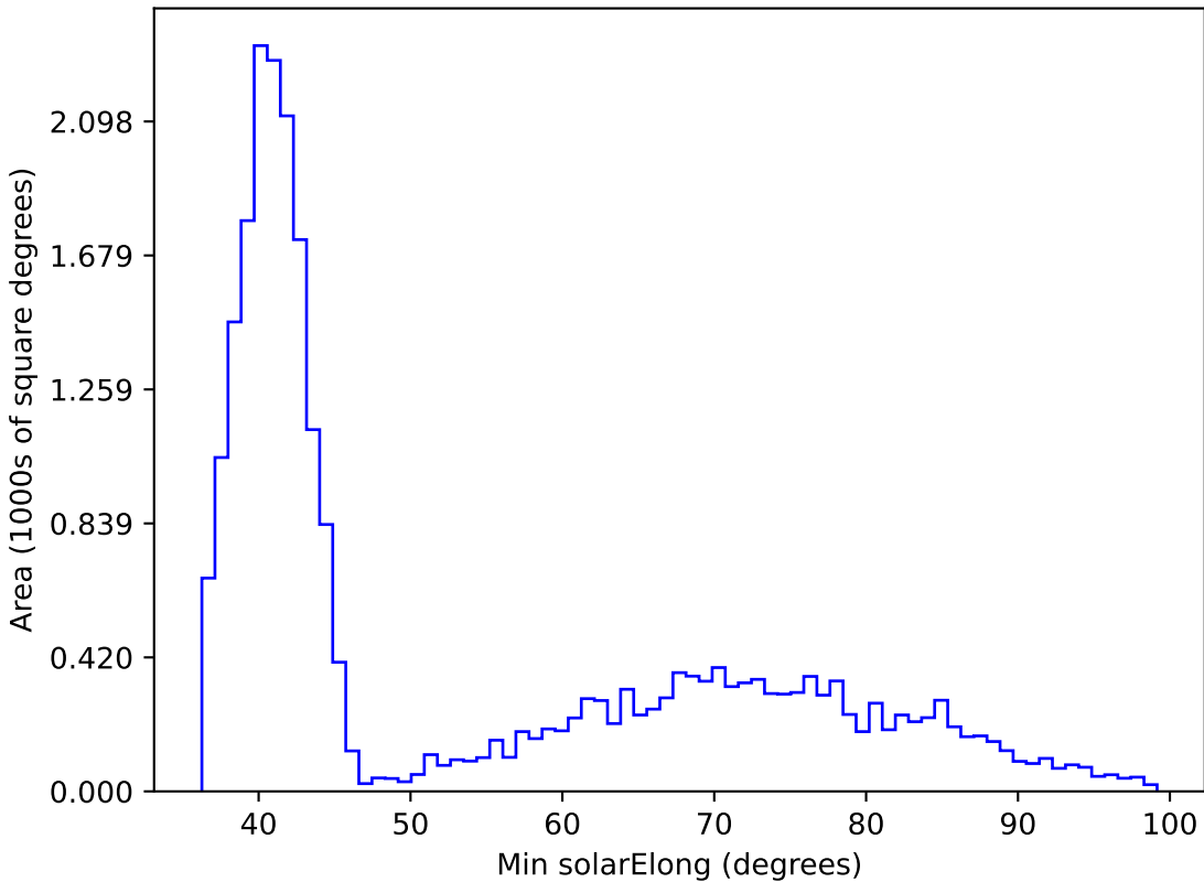
baseline_v3.3_10yrs All sky i band: Min solarElong
