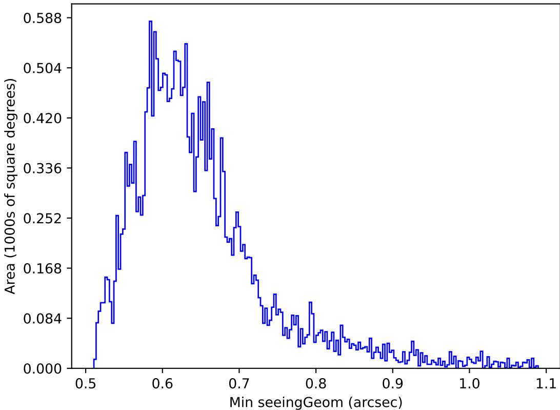
baseline_v3.3_10yrs Yr 1 z band: Min seeingGeom
