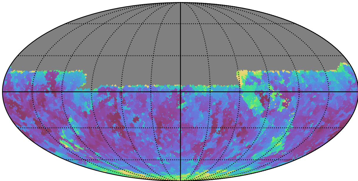
baseline_v3.3_10yrs Yr 1 y band: Min seeingGeom
