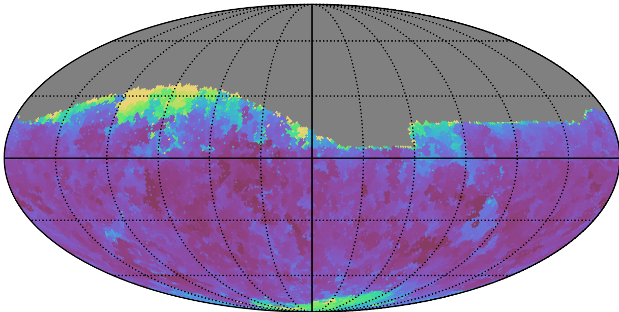
baseline_v3.3_10yrs Yr 1 r band: Min seeingGeom
