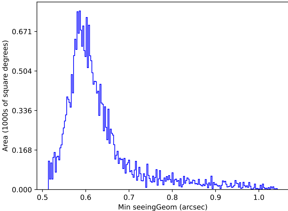
baseline_v3.3_10yrs Yr 1 i band: Min seeingGeom
