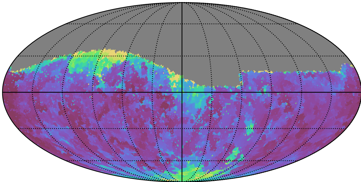
baseline_v3.3_10yrs Yr 1 g band: Min seeingGeom
