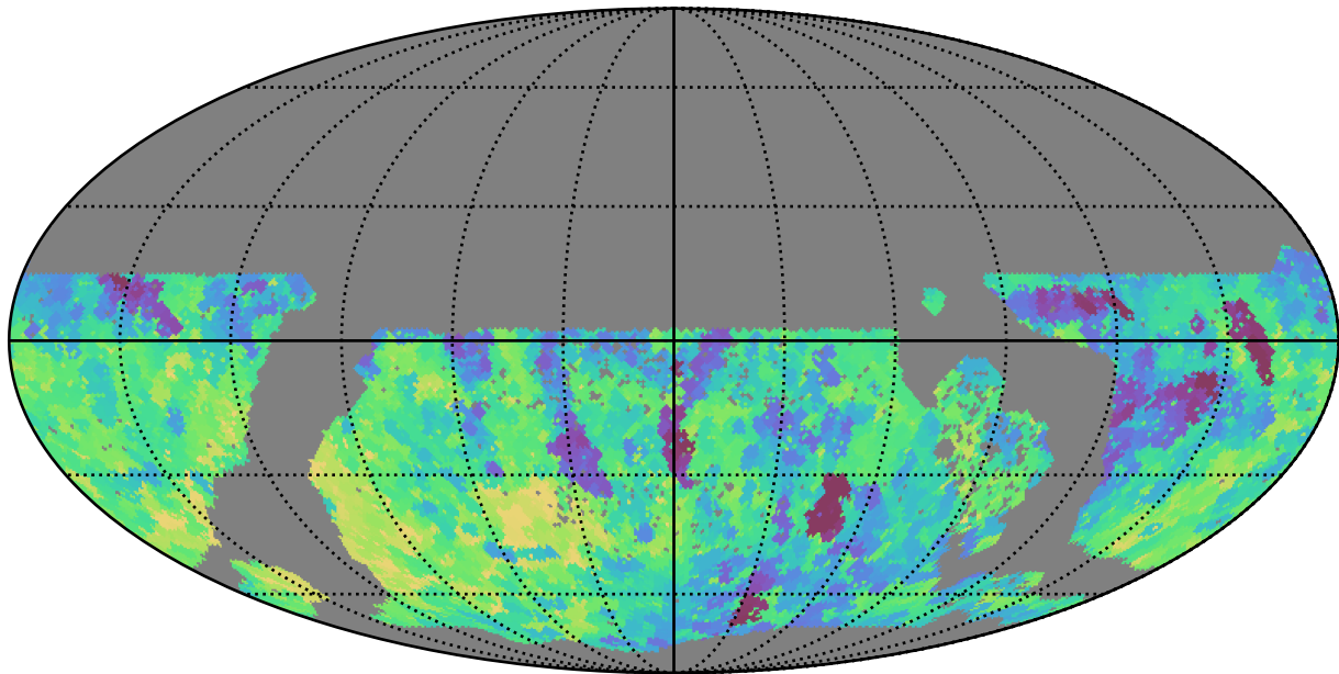
baseline_v3.3_10yrs WFD z band: Min saturation_mag
