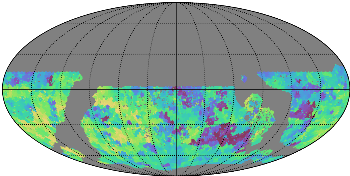
baseline_v3.3_10yrs WFD y band: Min saturation_mag
