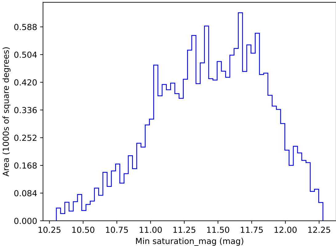
baseline_v3.3_10yrs WFD u band: Min saturation_mag
