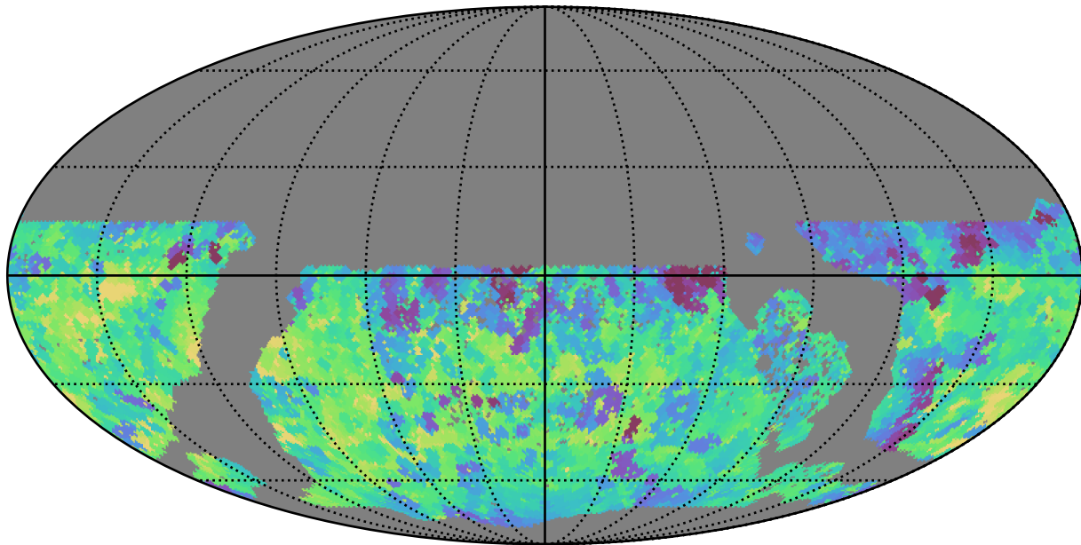
baseline_v3.3_10yrs WFD r band: Min saturation_mag
