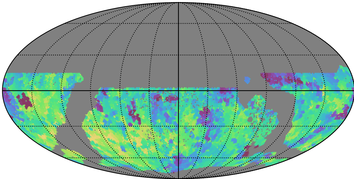
baseline_v3.3_10yrs WFD i band: Min saturation_mag
